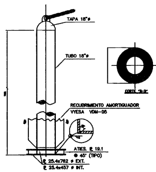
DETALLE 3.- CAMISA DE RECURRIMIENTO VIESA VDM-05
