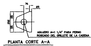
PLANTA CORTE A-A
