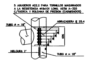
D-2 ELEVACION TUBO 18"
