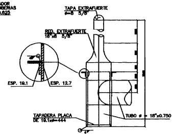
D-4 GUIA DE ACOPLAMIENTO
