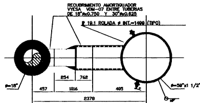
PLANTA CORTE B-B
