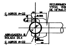
PLANTA CORTE B-B
