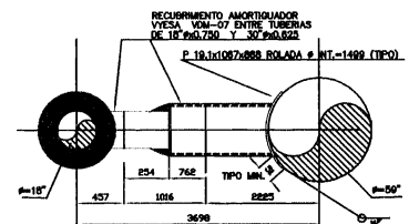
PLANTA CORTE A-A
