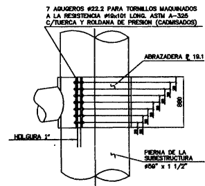
DETALLE 5.- ELEVACION DE ABRAZADERA
