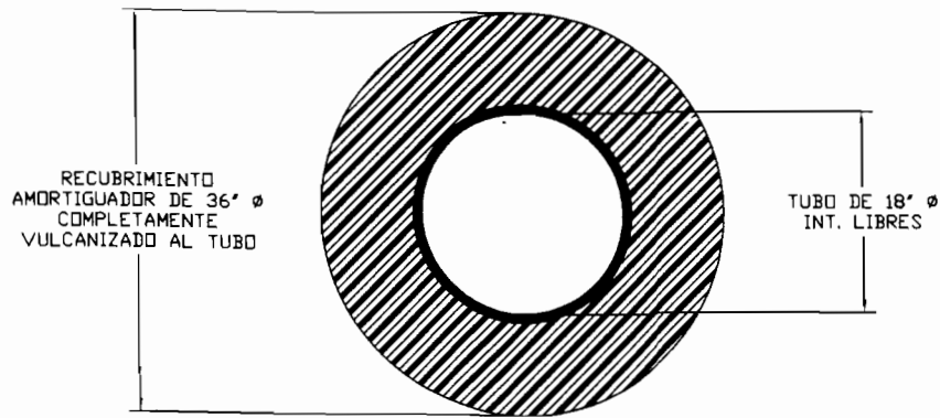
SECCION "X-X" ESCALA : 1:20
