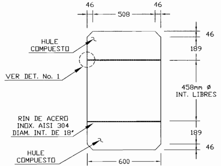
SECCION "A-A"
